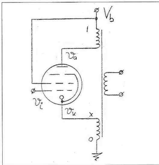
fig.28 Super-ultra-lineaire schakelwijze.
